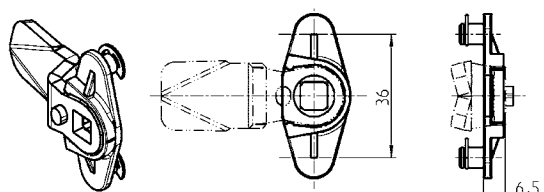
Propulsore per aste in zama zincata, seeger in acciaio zincato
